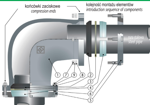
Łącznik zaciskowy flanszowy Flange compression
